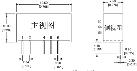
封装尺寸图
