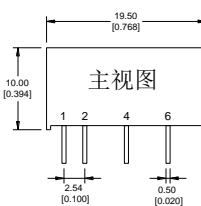
封装尺寸图
