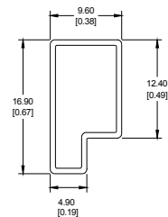
注： 单位 (Unit) : mm [inch] 未注明公差: x.x±0.5mm [x.x±0.020inch] 0.x±0.2mm [x.x±0.008inch] 管长: 220mm [8.66inch] 包装数量: 17pcs 内盒: 235*160*82mm 包装: 9管*6层 外箱: 335*225*280mm 包装: 6盒*1箱
