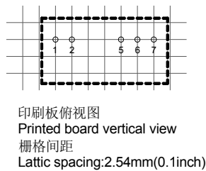
建议印刷板图
