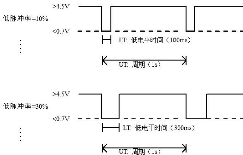
图5 PM2.5输出波形图
