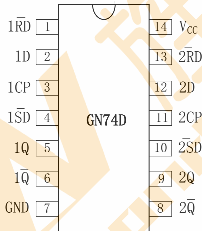
图 3、引脚排列图
