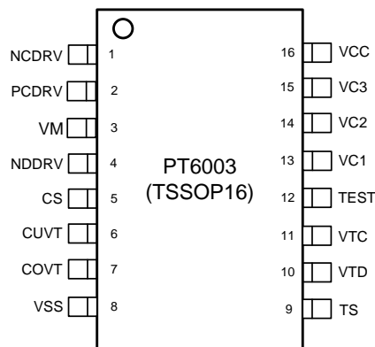
图 3. 管脚定义图
