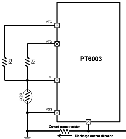
图 5. 温度检测电路
