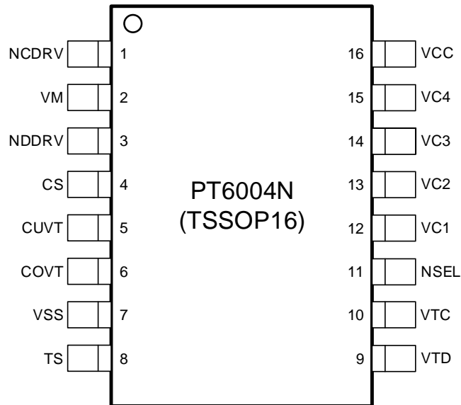
图 3. 管脚定义图
