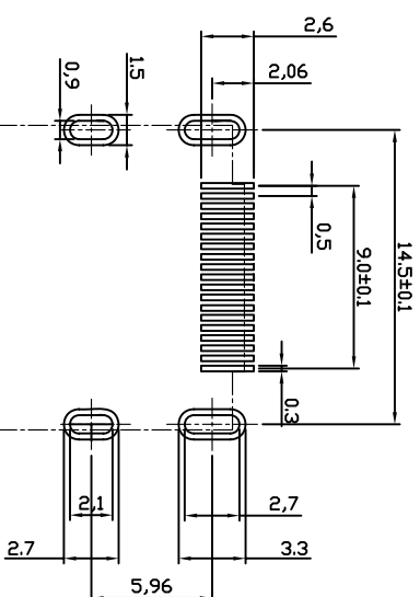
P.C.B LAYOUT(±0.05)
