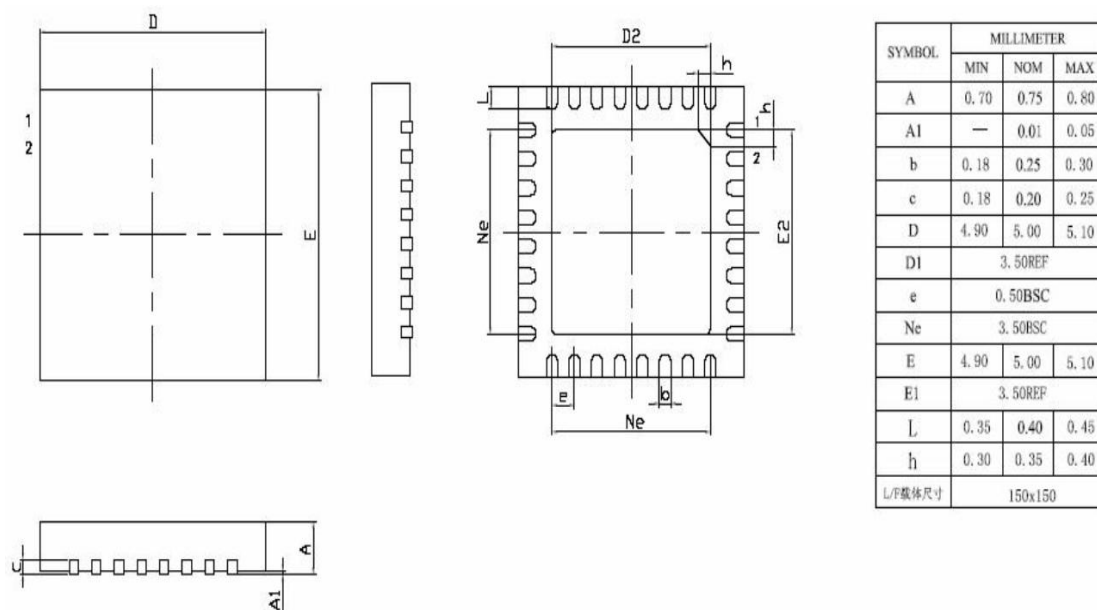
图 7 QFN32 封装尺寸
