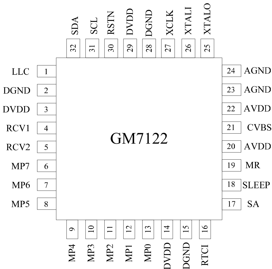
图 1 QFN32 管脚说明
