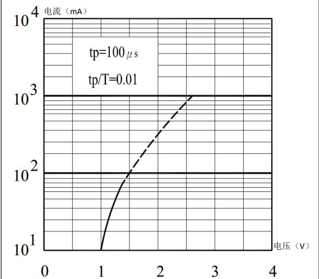
正向电流与正向电压的关系
