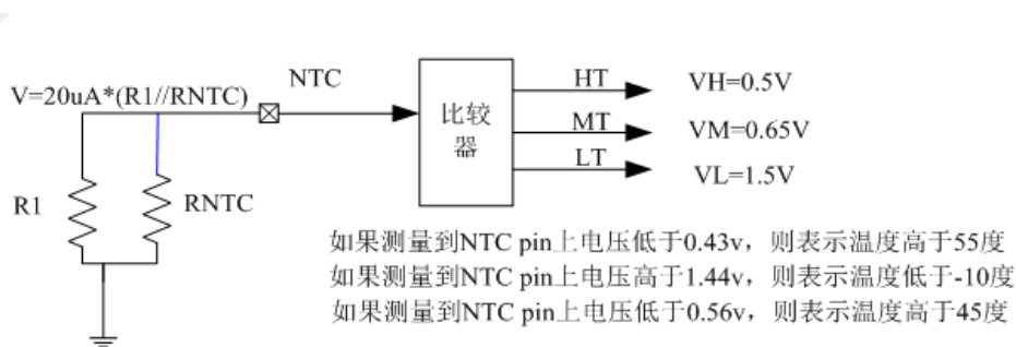
图 4 电池 NTC 比较
