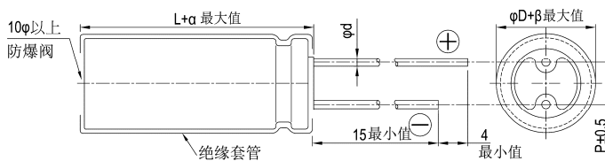
寸法图
