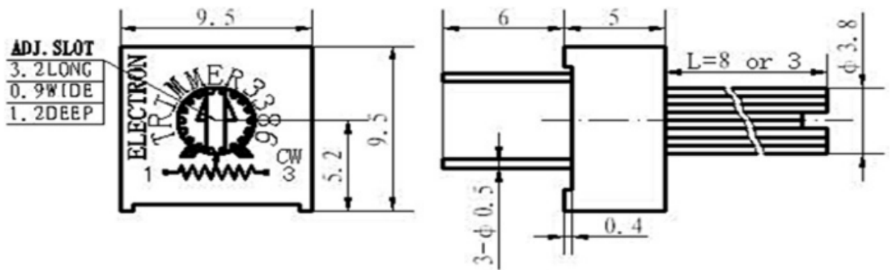
3386P型
