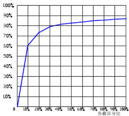
效率曲线
