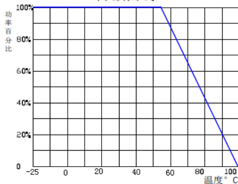
降额曲线
