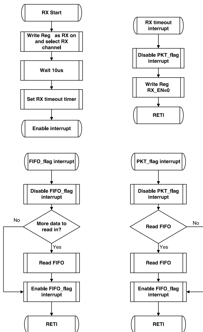
接收流程图
