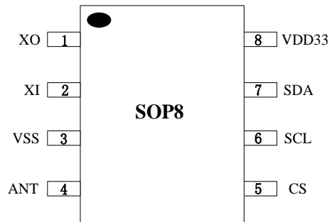
图5.1 RC808 引脚图
