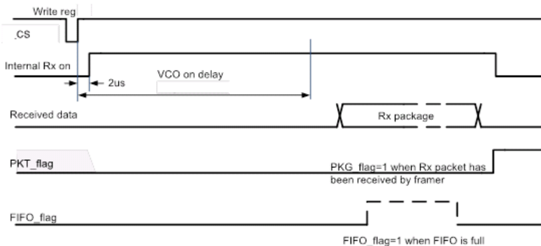
接收时序图
