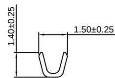
SEC:B-B
