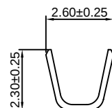
SEC:A-A
