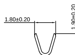
SEC:A-A
