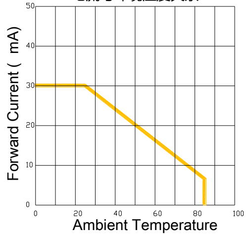
电流与环境温度关系
