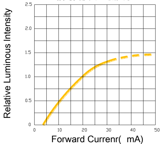
Relative Luminous Intensity vs. Forward Current 相对亮度与电流关系
