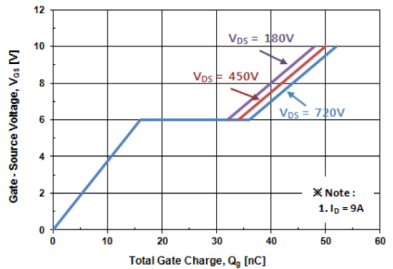
Fig. 6 V_{GS} - Q_G
