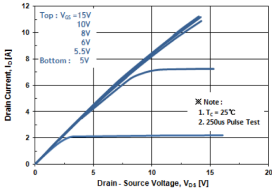
Fig. 1 I_D - V_{DS}
