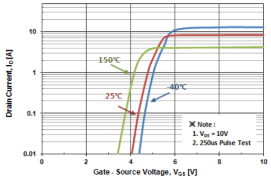
Fig. 2 I_D - V_{GS}
