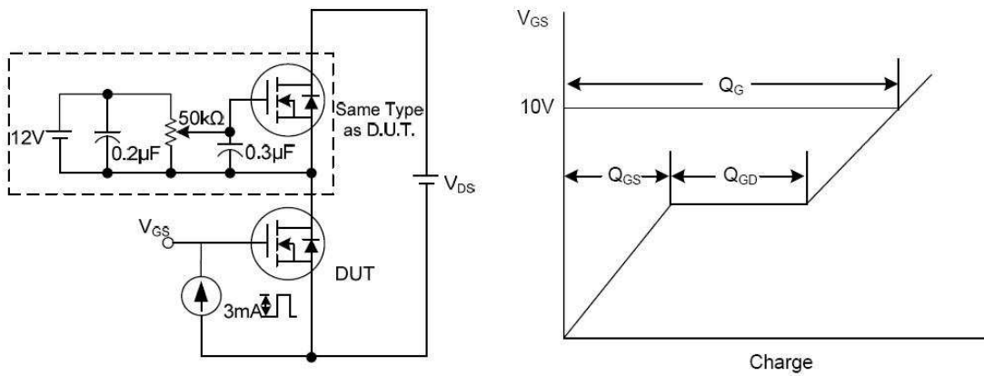
图11. 栅电荷测试
