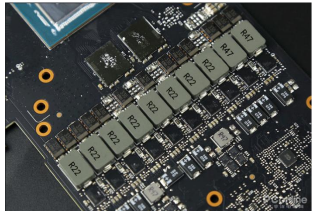
显示卡 (二)
