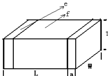
外形尺寸图:
