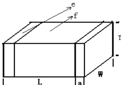
外形尺寸图:
