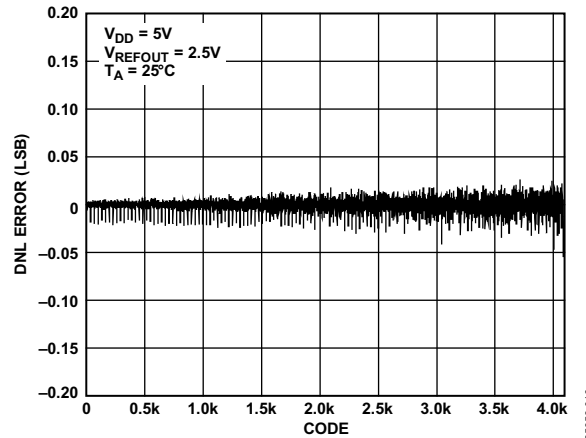
图15. DNL—AD5623R-5
