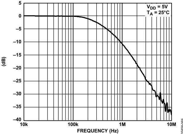
图47. 乘法带宽
