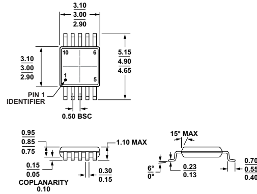
图64. 10引脚超小型封装[MSOP]
