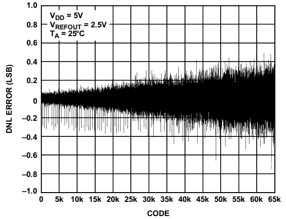
图13. DNL—AD5663R-5
