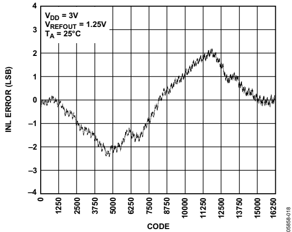
图17. INL—AD5643R-3
