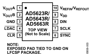
图3. 引脚配置
