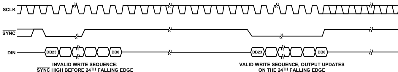
图54. SYNC中断设置
