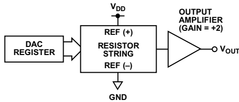
图49. DAC结构
