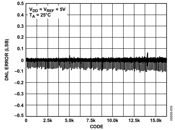
图8. DNL—AD5643R, 外部基准电压源
