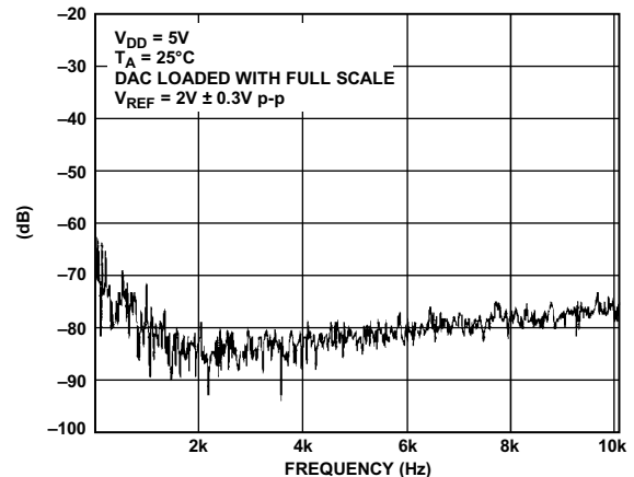
图45. 总谐波失真
