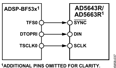
图56. AD5623R/AD5643R/AD5663R与Blackfin ADSP-BF53X接口
