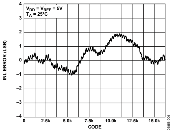
图5. INL—AD5643R, 外部基准电压源
