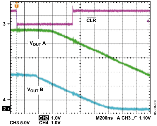
图48. CLR脉冲激活时间
