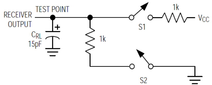
图 4. 接收时间测试电路
