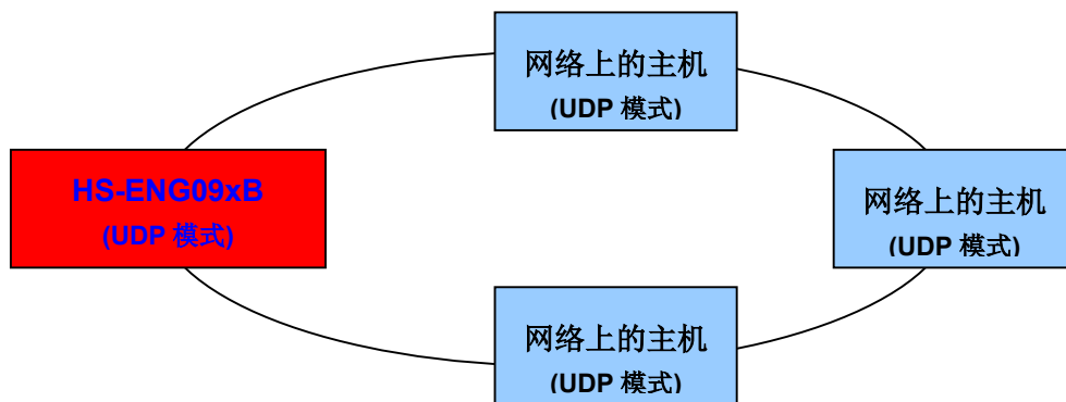
图 4.7 HS-ENG09xB 工作在 UDP 模式的逻辑图
