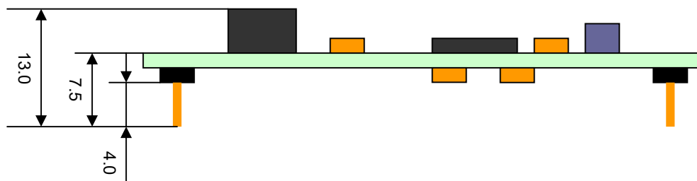
图2.2 HS-ENG092B尺寸图
