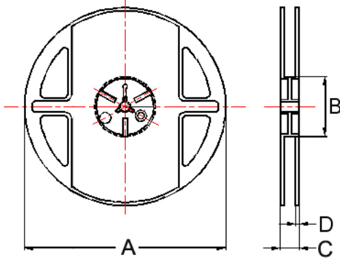
Reel Dimensions
