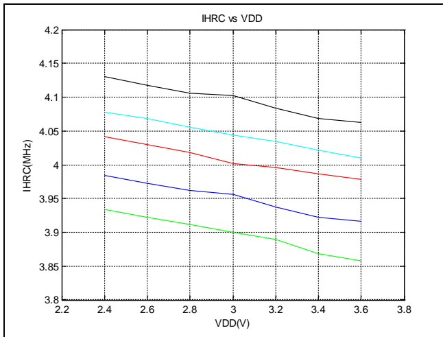
图4. IHRC 电压特性曲线
