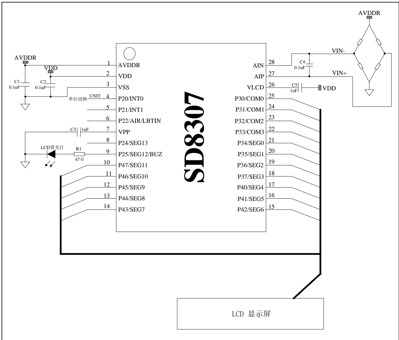
图 3. 典型应用图
