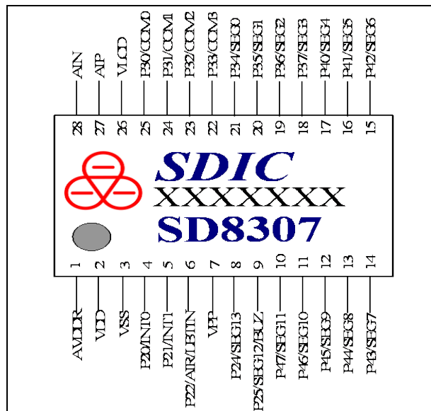
图 1. 管脚图
