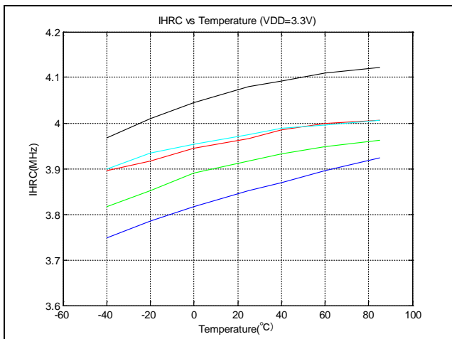
图6. IHRC 温度特性曲线
