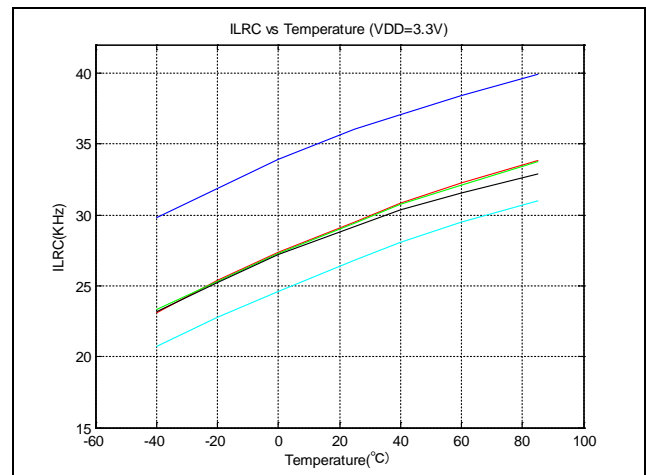
图7. ILRC 温度特性曲线
