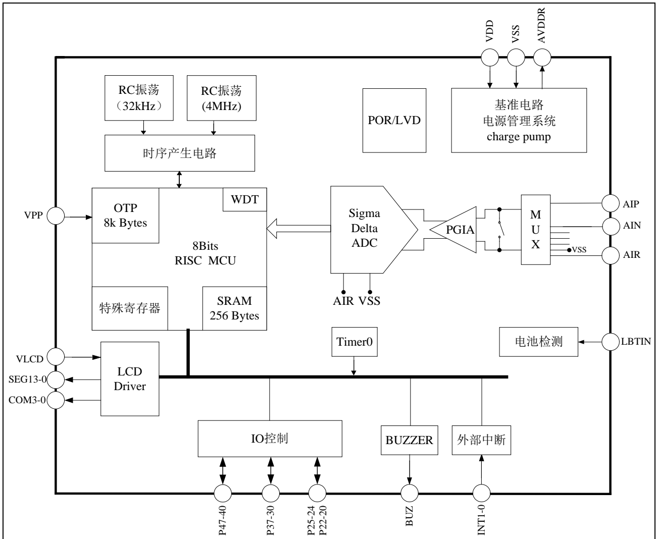
图2. 功能框图
