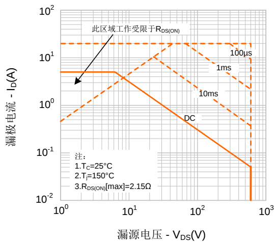
图9-1. 最大安全工作区域(SVF5N60F)
