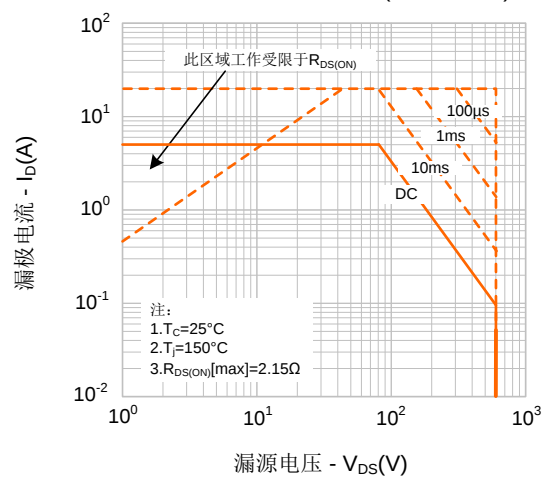
图9-2. 最大安全工作区域(SVF5N60D)
