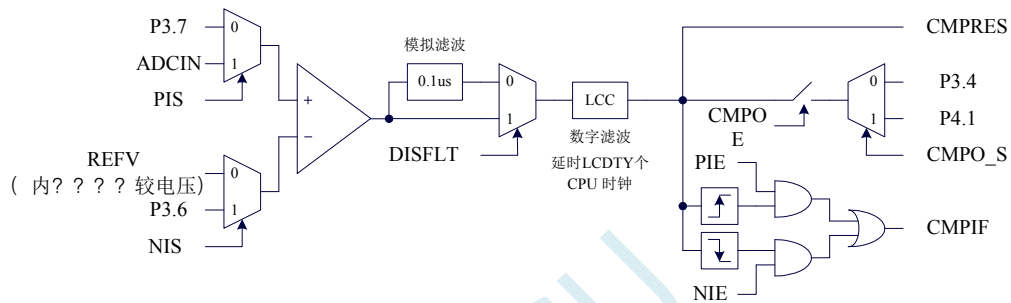
比较器内部结构
