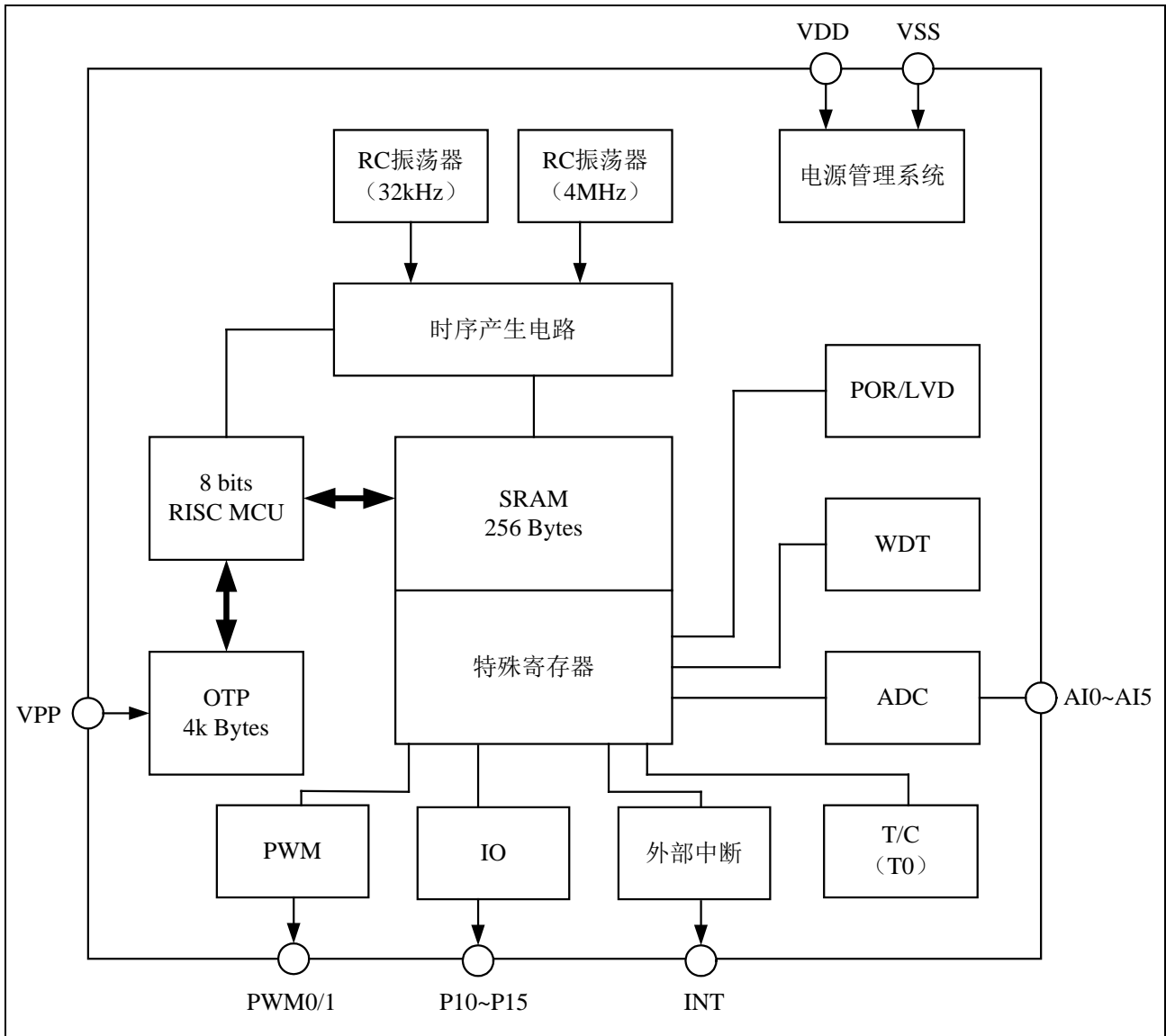
图2. 功能框图
