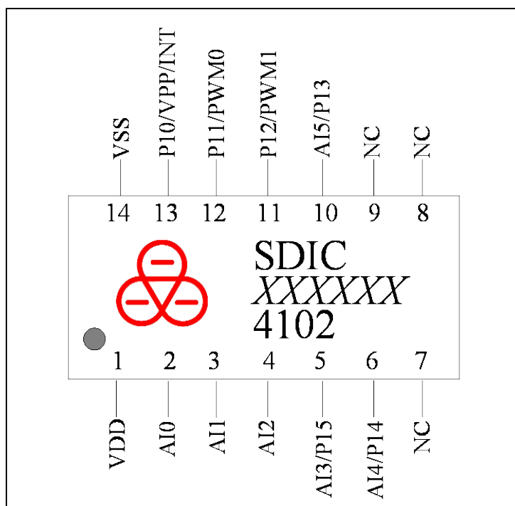
图 1. 管脚图
