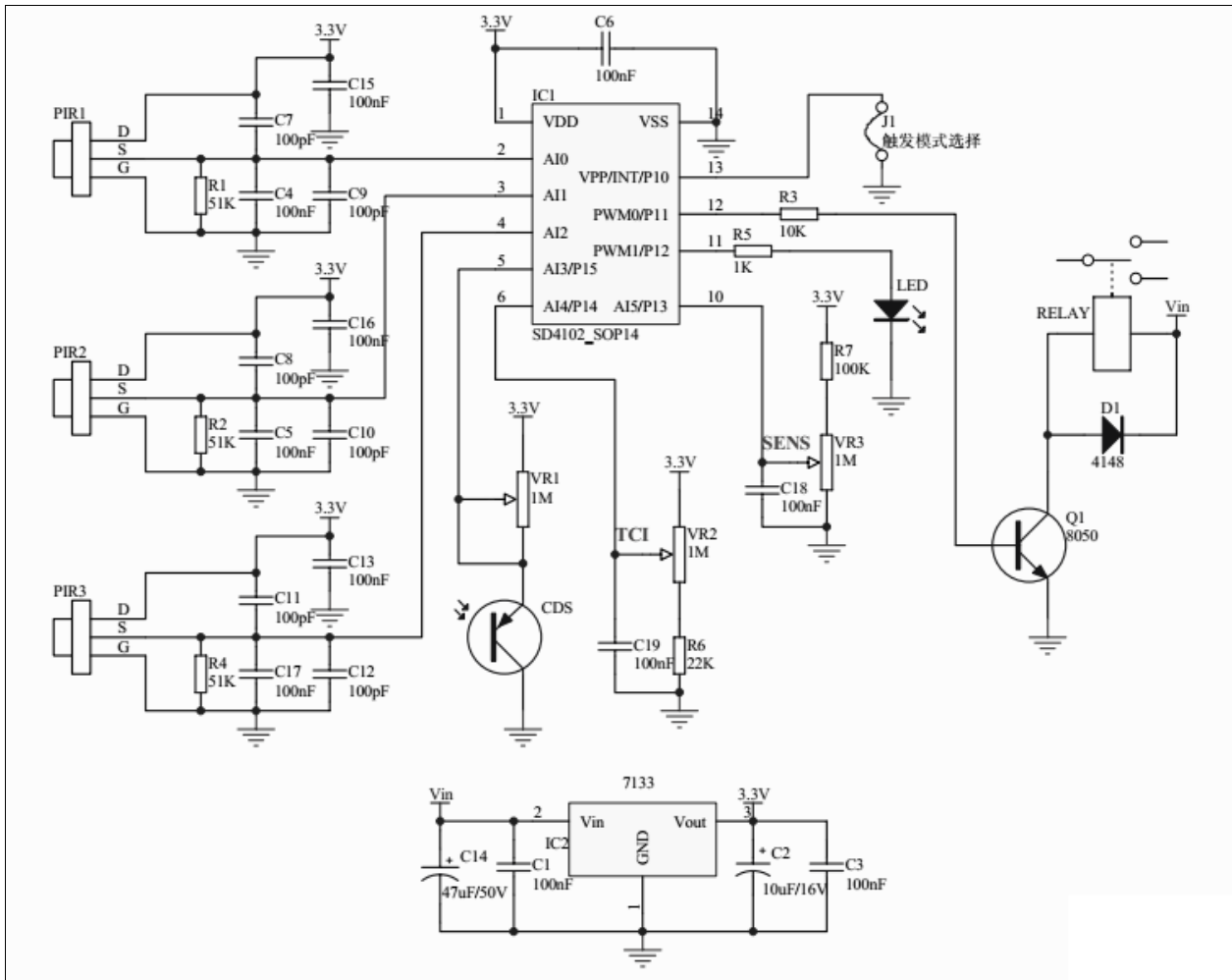
图 3. PIR 典型应用图
