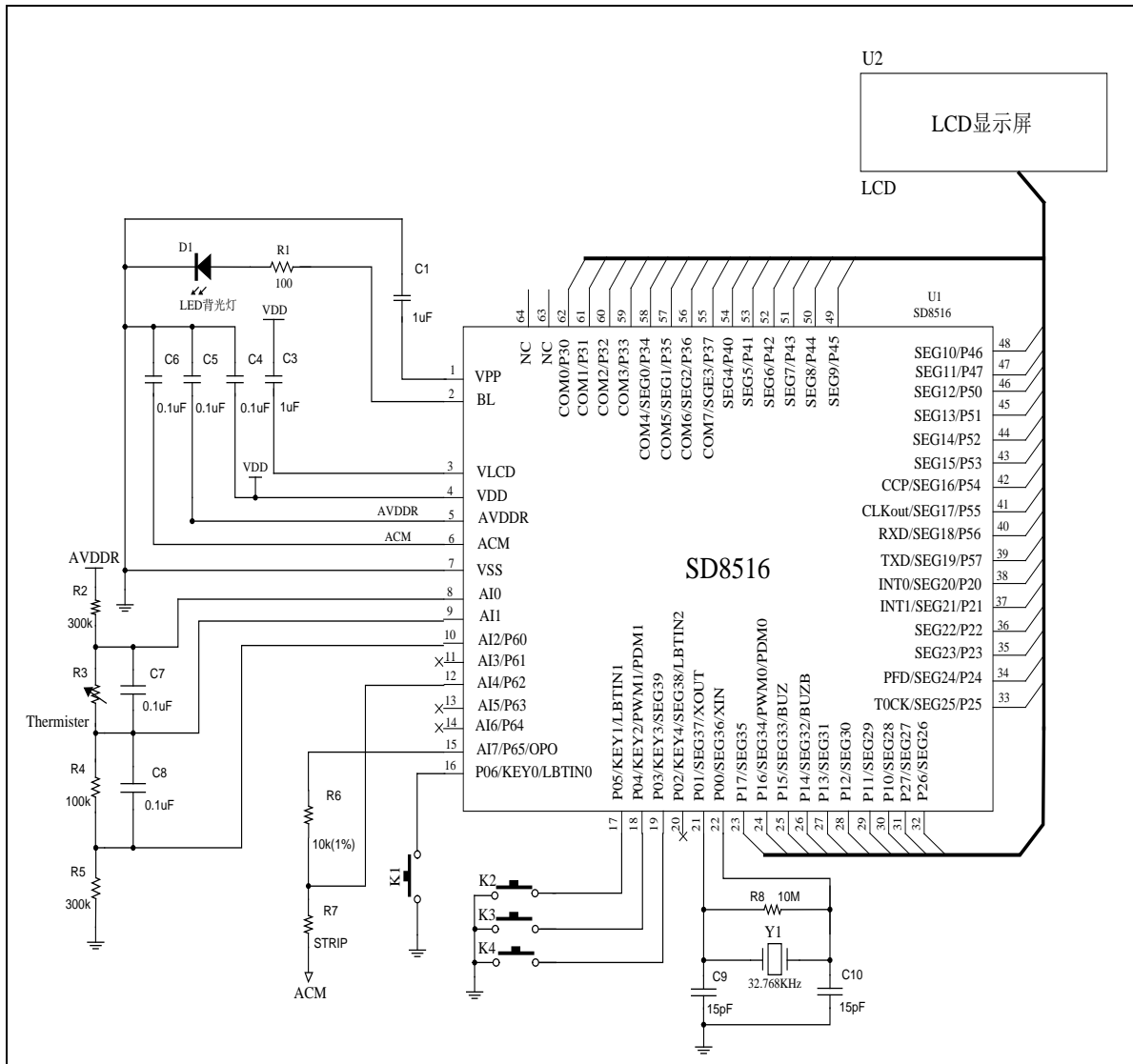
图 4.血糖仪
