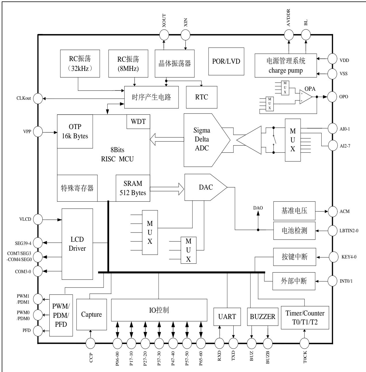
图 2. 功能框图
