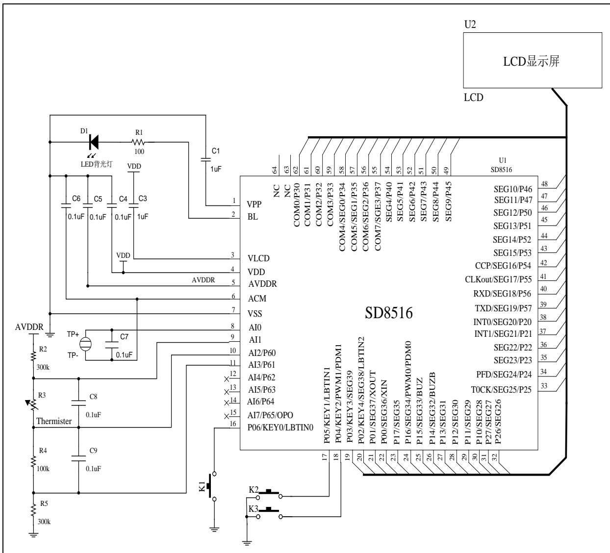
图 5. 红外测温
