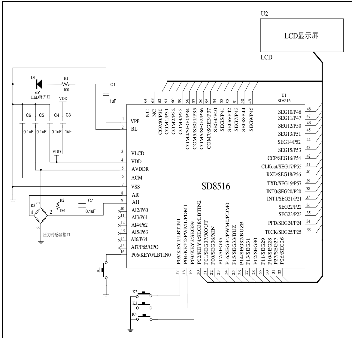
图 3. 电子秤
