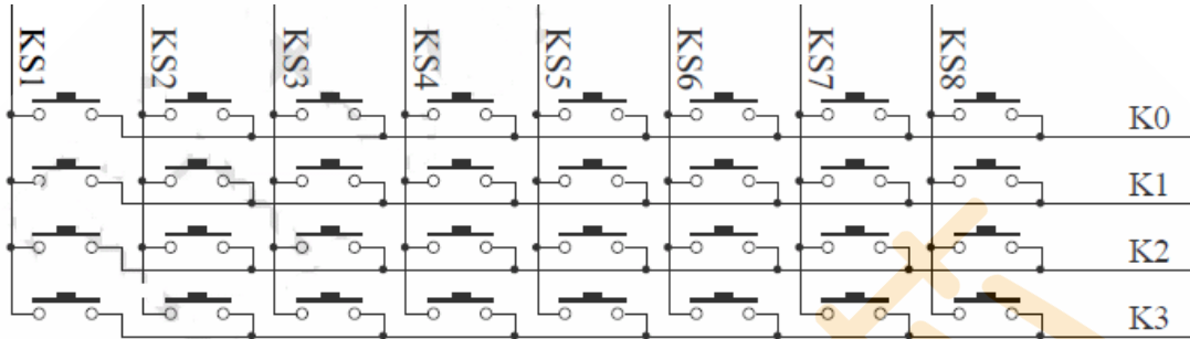
图 4、键扫矩阵
