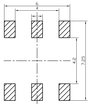
安装参考图
