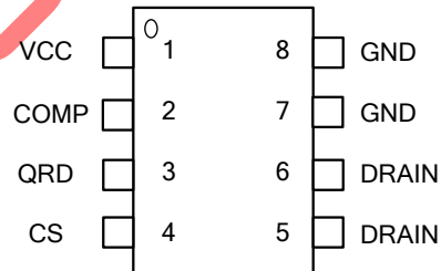
DIP-8
