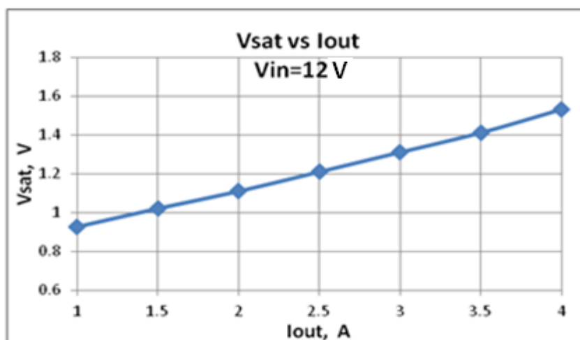
Fig.6. Vsat vs Iout
