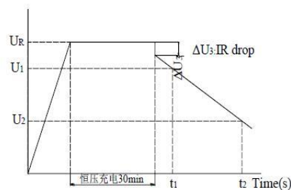
图 2. 充放电曲线图
