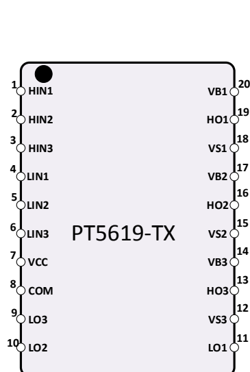
20-PIN TSSOP
