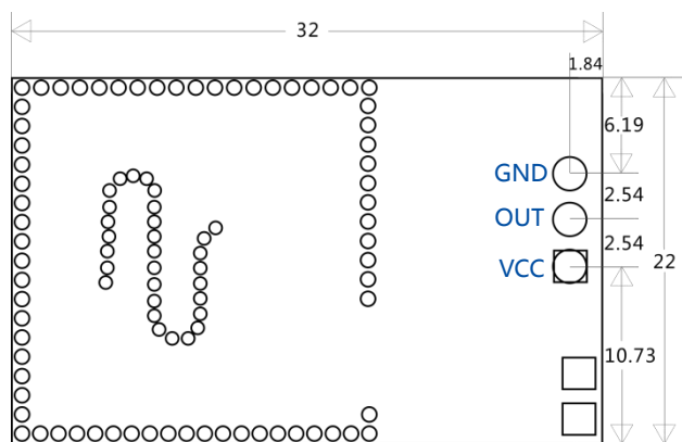
俯视图 (单位:mm)
