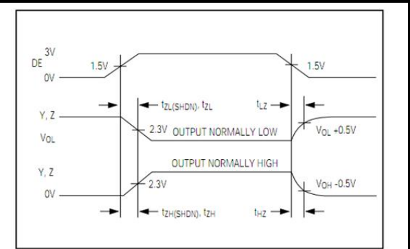
图 6 驱动器使能/禁能时序
