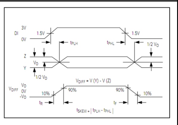
图 4 驱动器传播延迟
