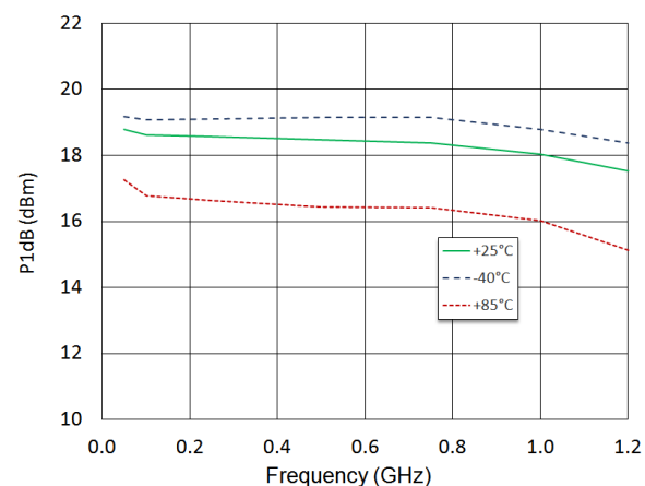
P1dB
