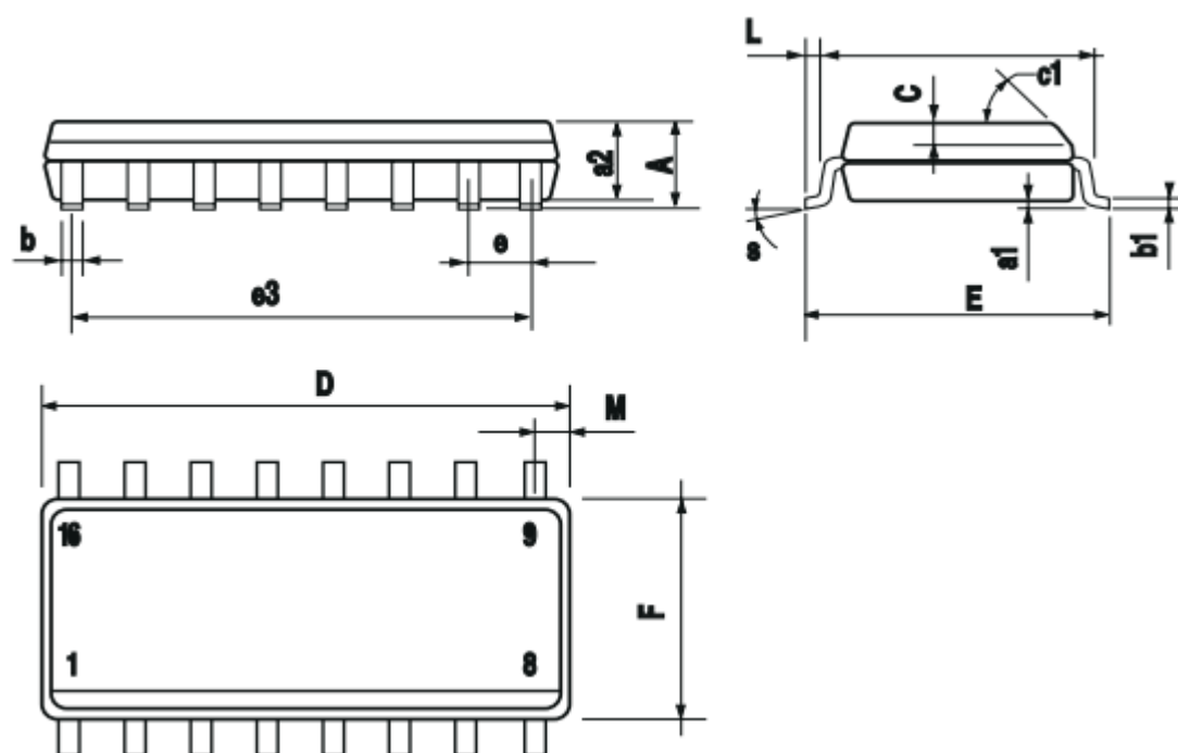
SOP16窄体
