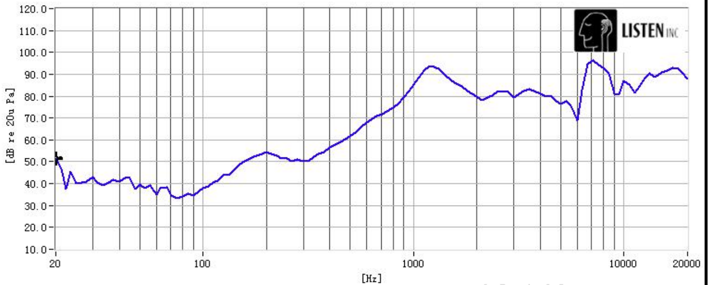
頻响曲线
