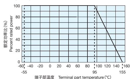
端子部温度 RK73H W3A2
