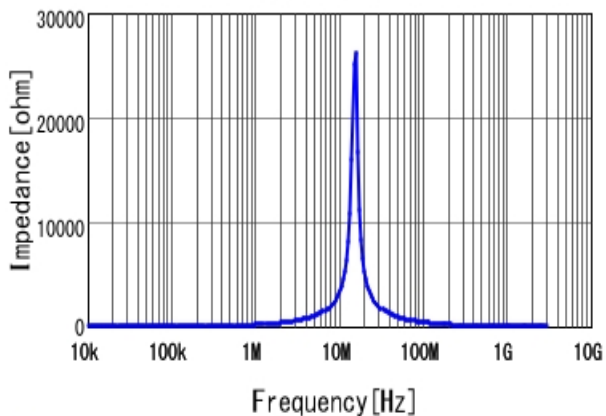
■ DEM8045Z-330M |Z|
