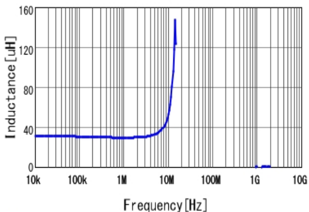
■ DEM8045Z-330M L
