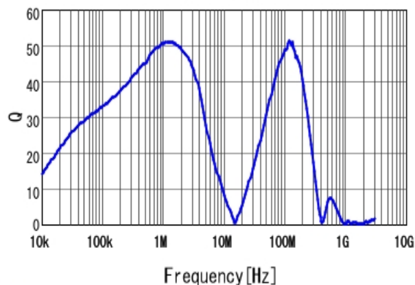
■ DEM8045Z-330M Q
