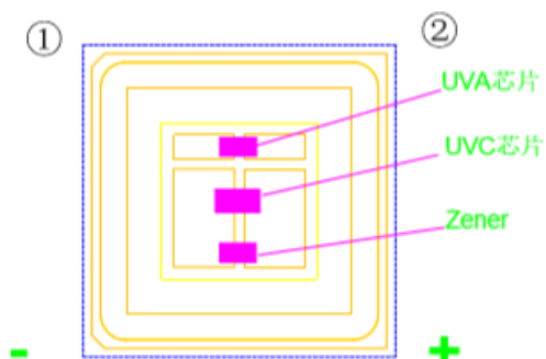
正面图
