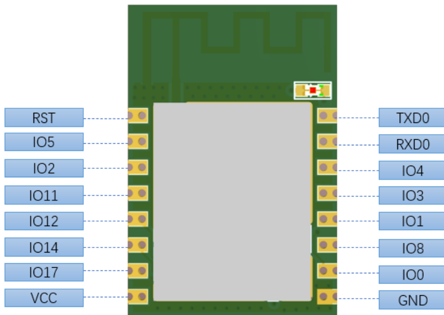
图 2.1 BL-62B 管脚示意图
