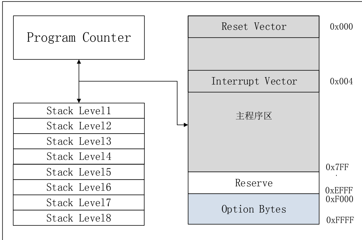
图 2-2 程序存储器
