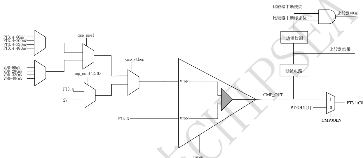
图2 模拟比较器框图
