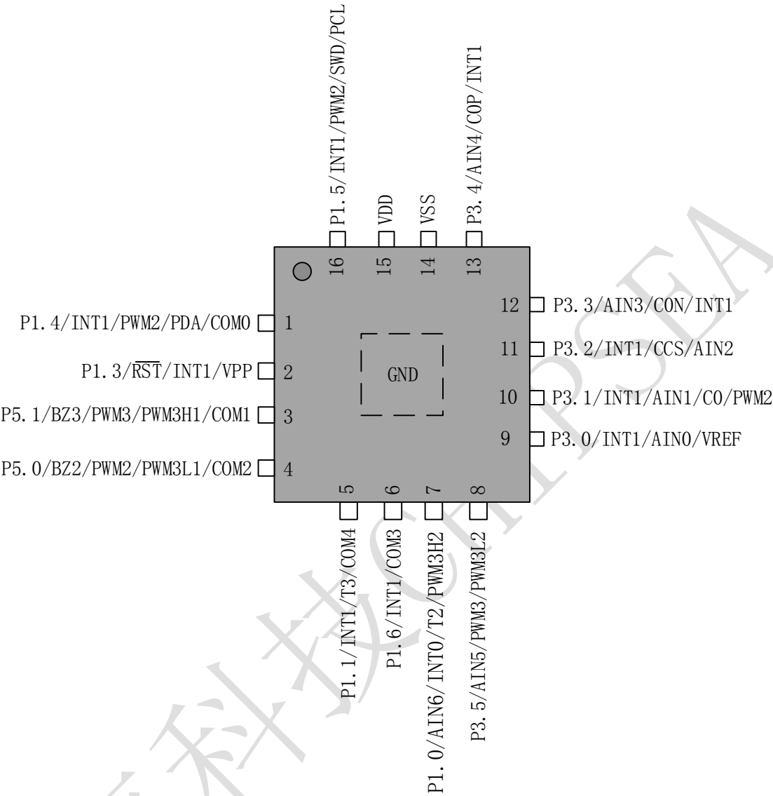
图 1-4 QFN16 PIN 配置图
