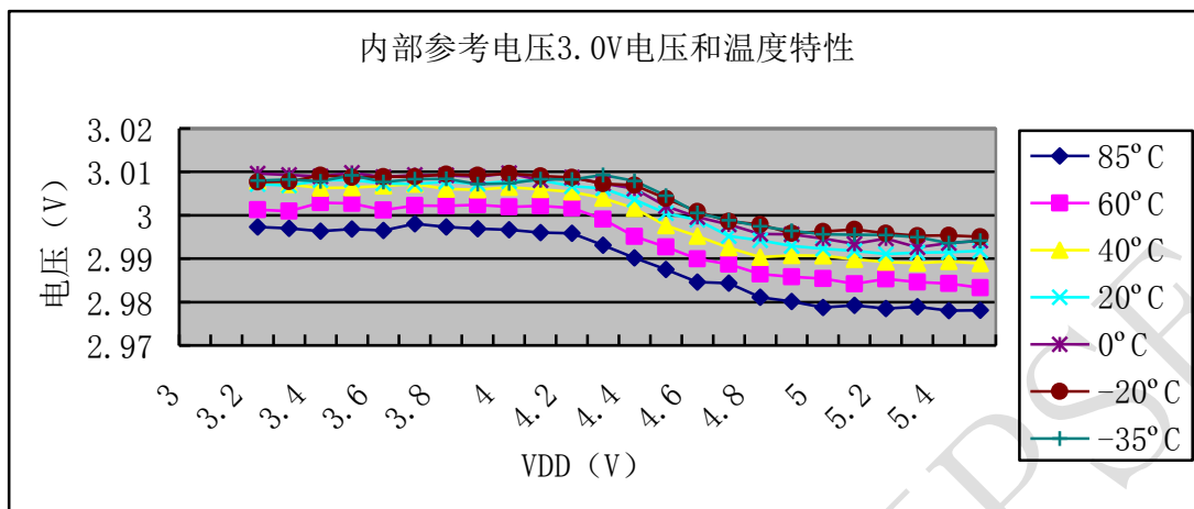
图 6-10 内置参考电压 3.0V 电压和温度特性
