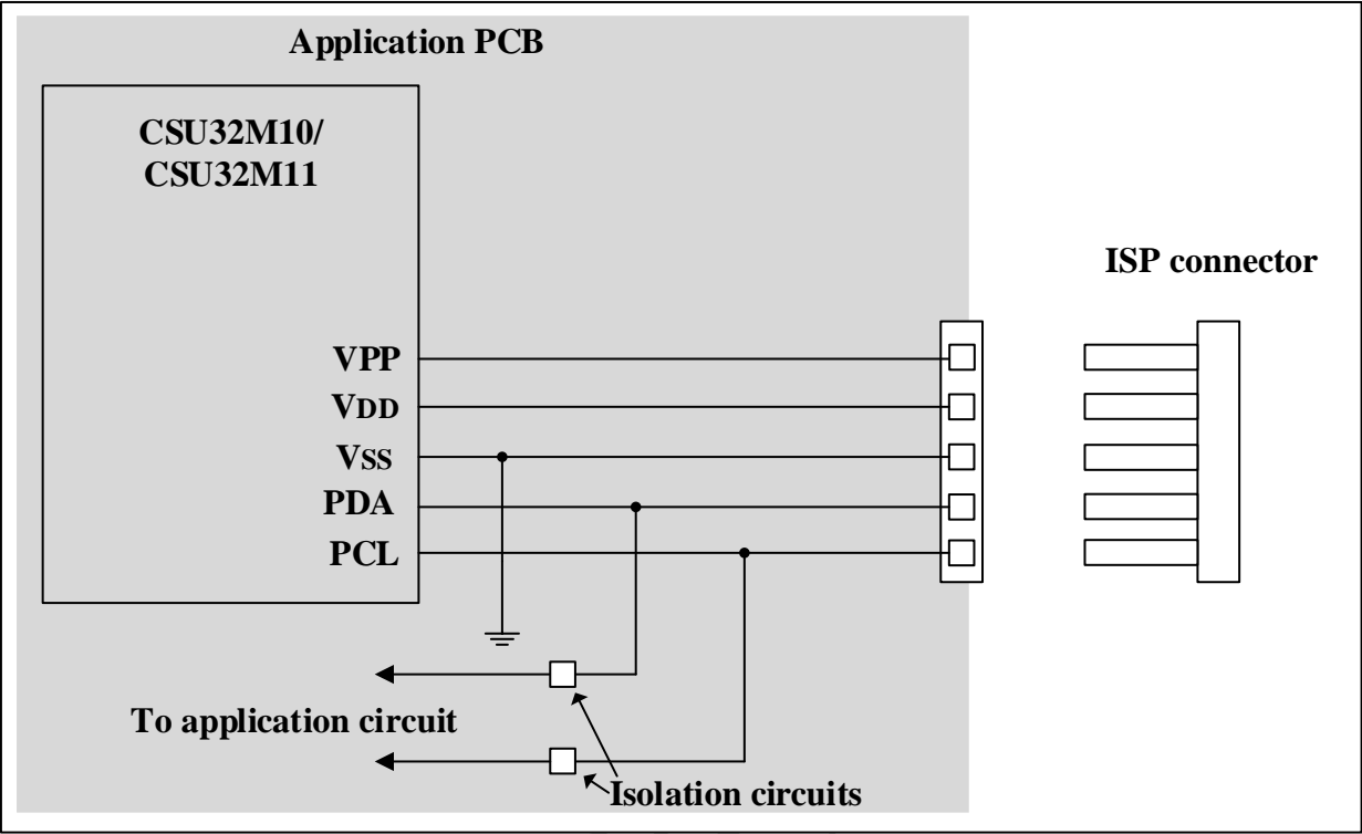
图 3-13 烧录器接口图
