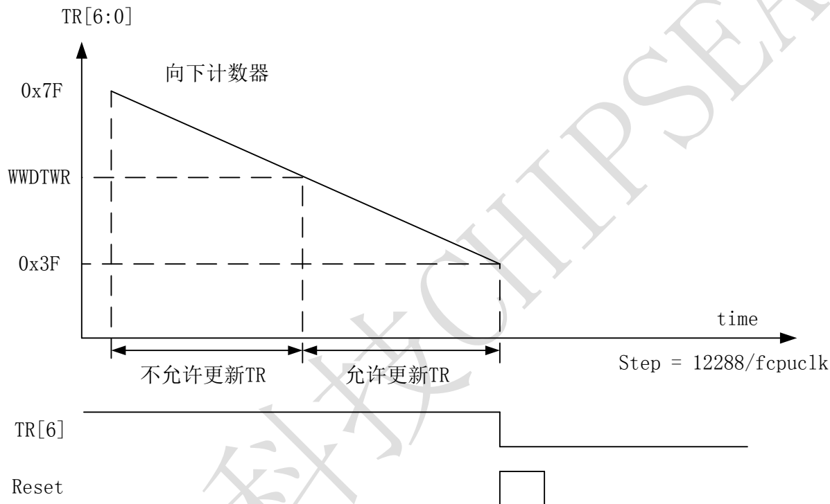
图 3-3 WWDT 时序图
