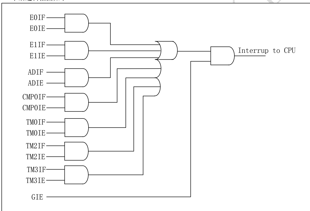
图 2-8 中断逻辑
