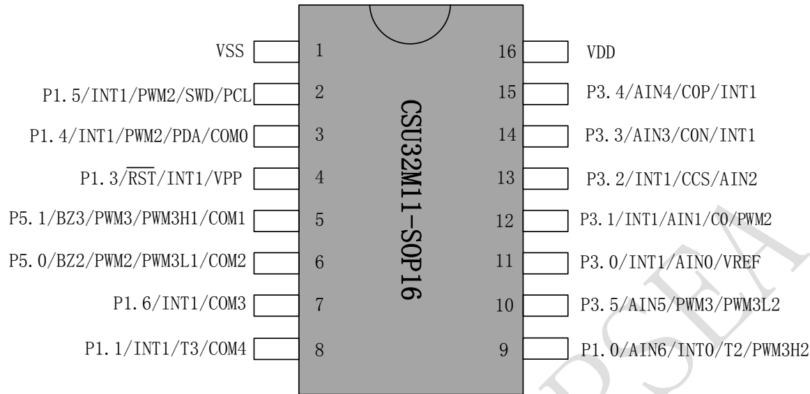
图 1-3 SOP16-2 管脚图
