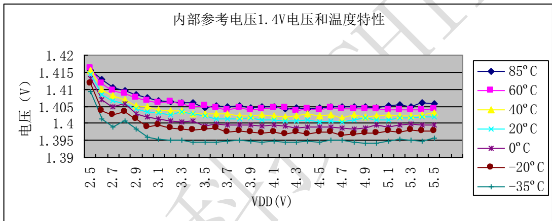
图 6-8 内置参考电压 1.4V 电压和温度特性
