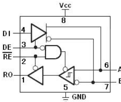
图2: GM75176E逻辑图
