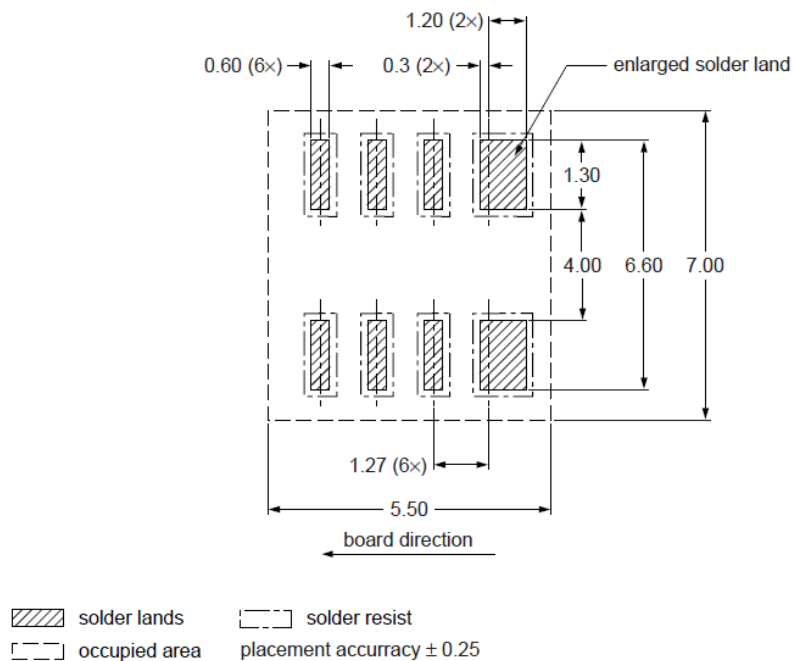
图 24. MSOP8/TSSOP8 PCB 引脚尺寸
