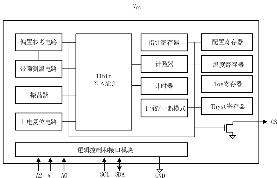
图 1. 芯片结构图
